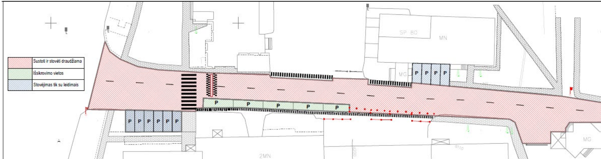
Priedas Nr. 2 „KPP priegų transporto priemonių stovėjimo schema“
